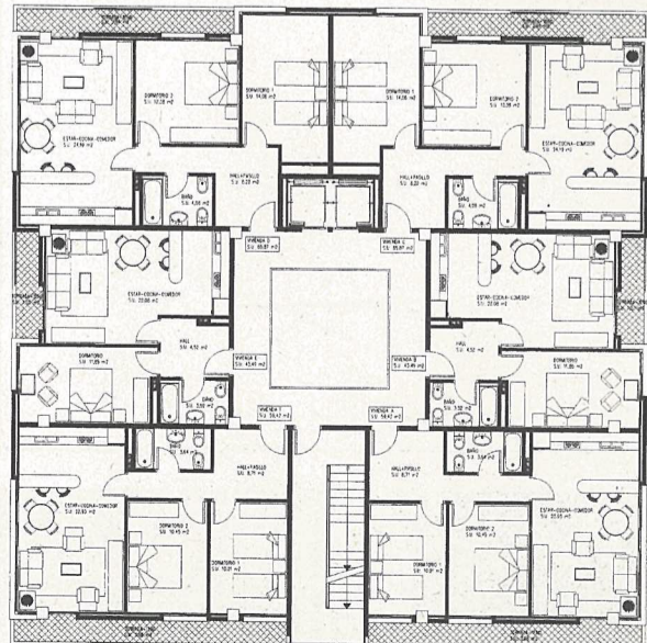
Planta, Sección, Axonom. y detalle fotograf. de VPO en Calahorra
