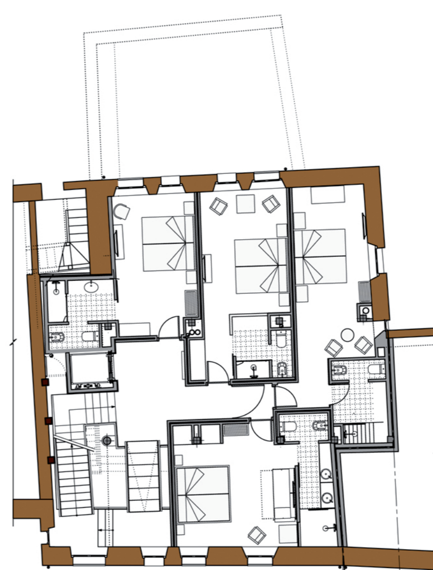
PLANTA PRIMERA Esc: 1/150
