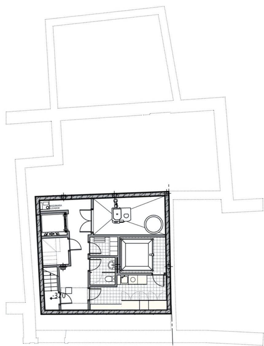
PLANTA SÓTANO Esc: 1/150
