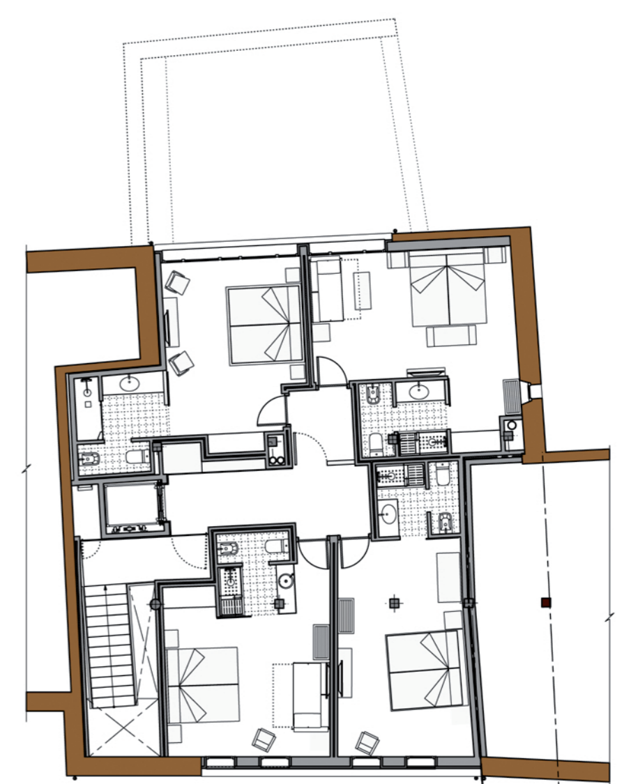
PLANTA SEGUNDA Esc: 1/150
